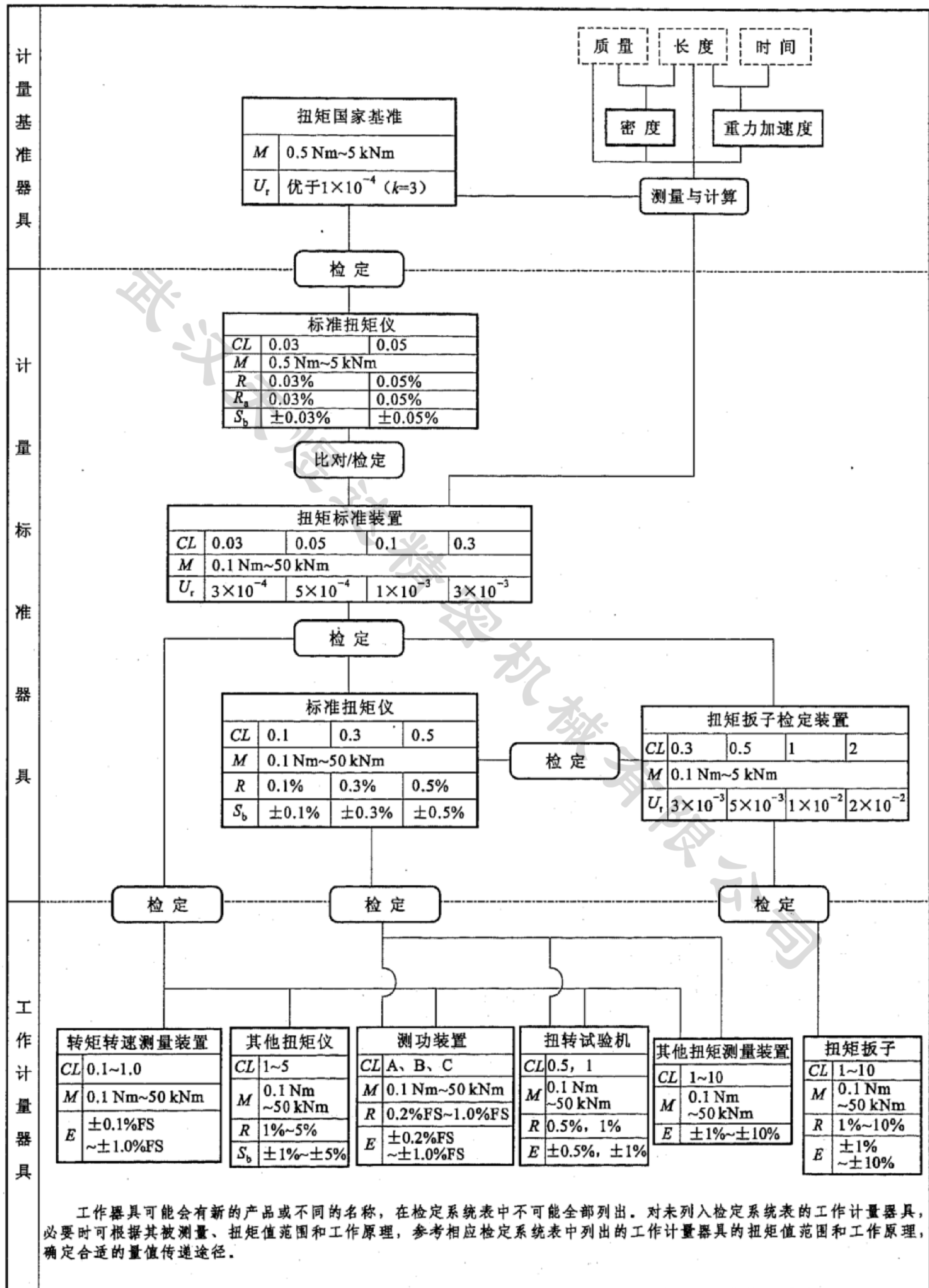
扭矩计量器具检定系统框图
